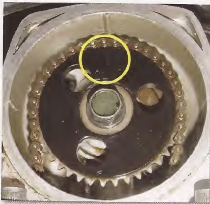
Toma de tiempo mecánico en motor horizontal
